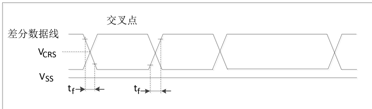
图15 USB2 时序：数据信号上升和下降的时间定义
